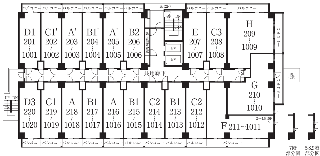
[ 2 ~ 10 階 平面 図 ]
