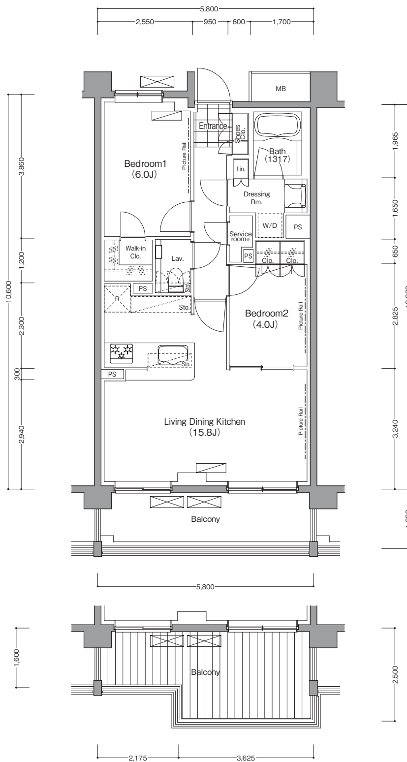
1階部分図
