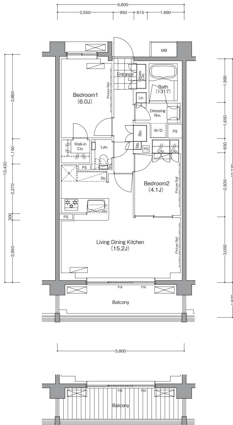
1階部分図
