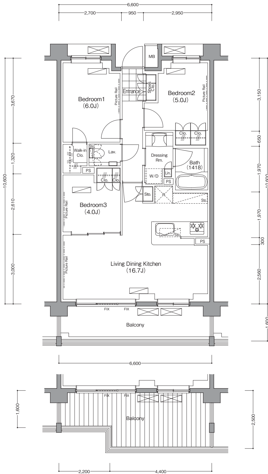
1階部分図
