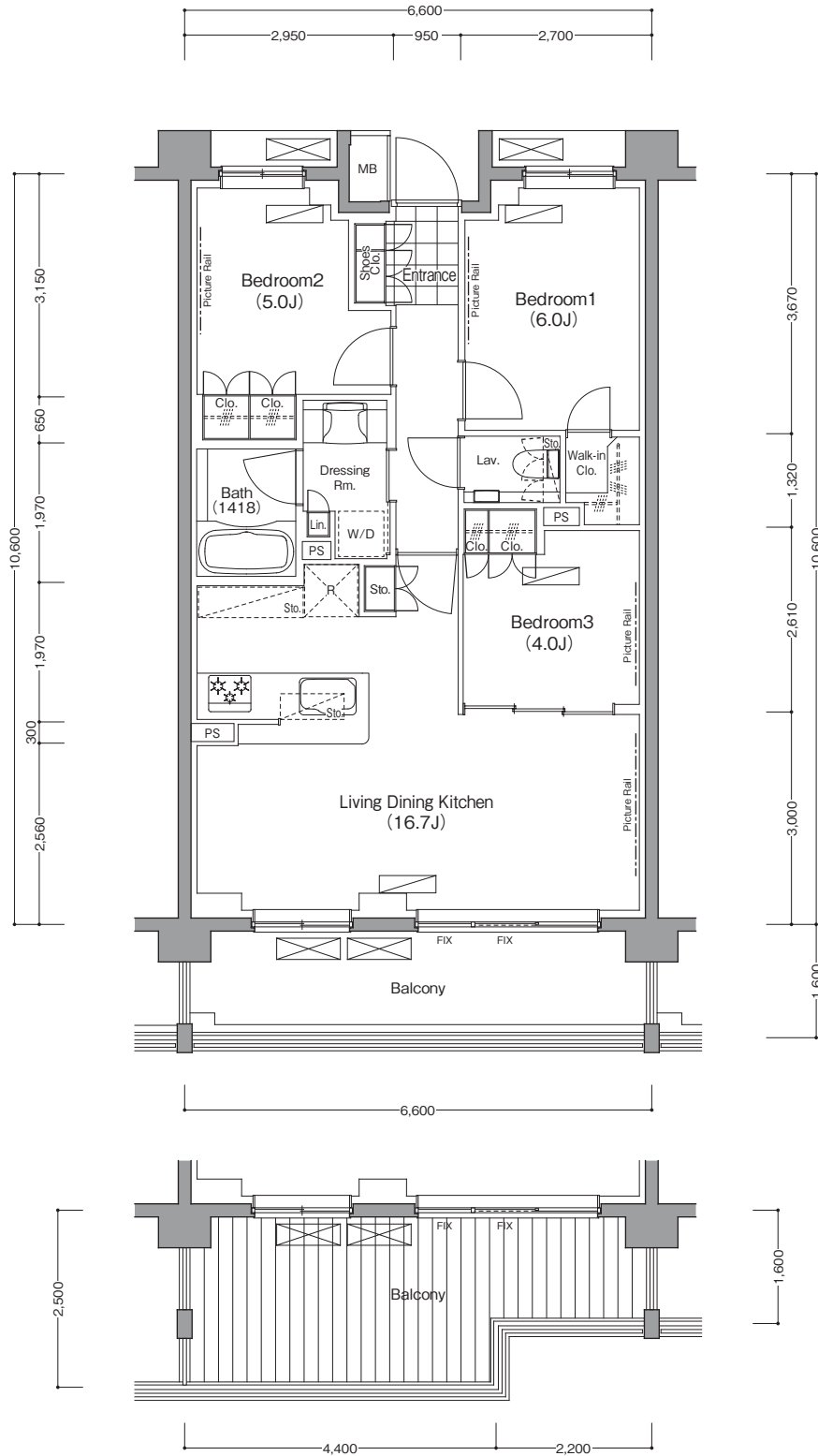
1階部分図
