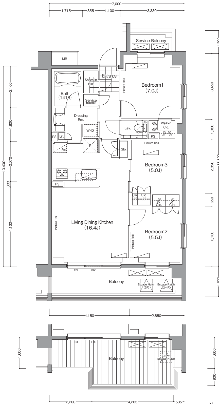
1階部分図
