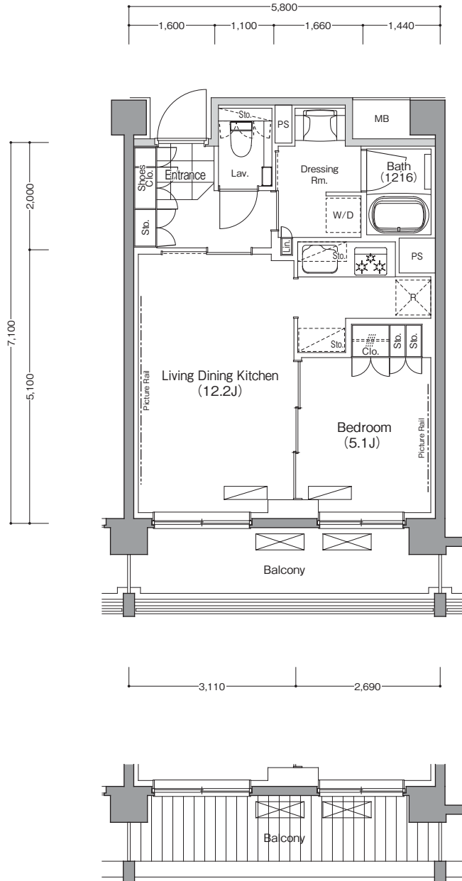
1階部分図
