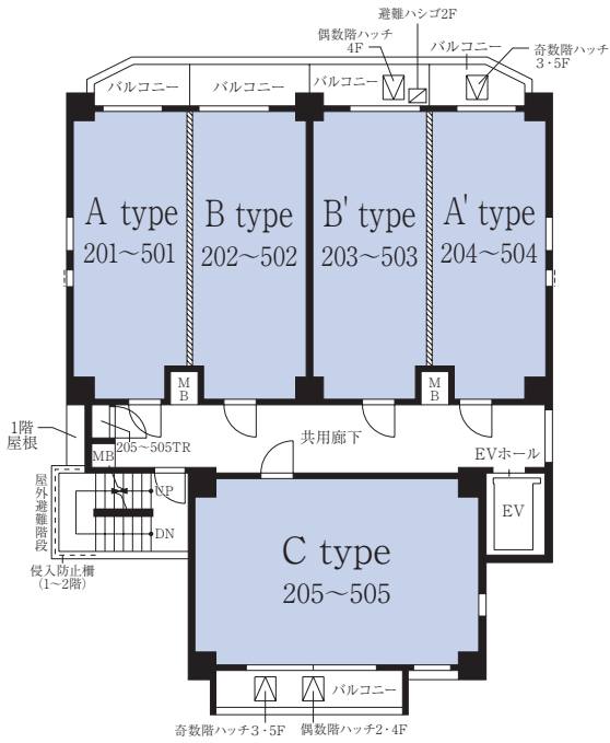
【2~5F平面図】
