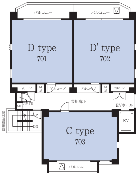
【7F平面図】
