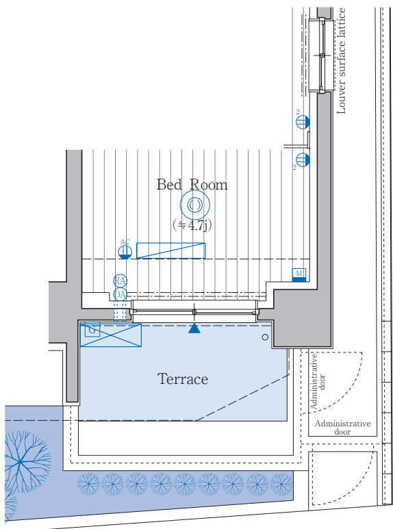
【1F部分図】
