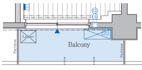
【2F部分図】
