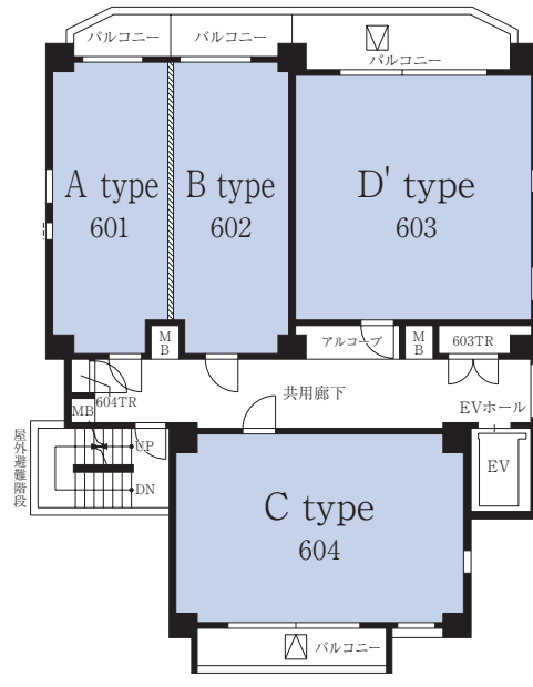
【6F平面図】
